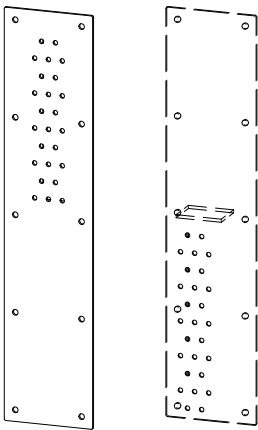
Grille phonique Rivetée, en acier inoxydable Déflecteur anti-intrusion
