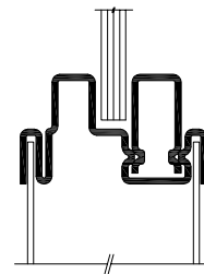
Moulures SI Verre 1/4" max.
