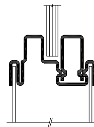
Moulures SI Verre 1/4" max.
