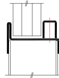
Moulures TH Verre 1" max.
